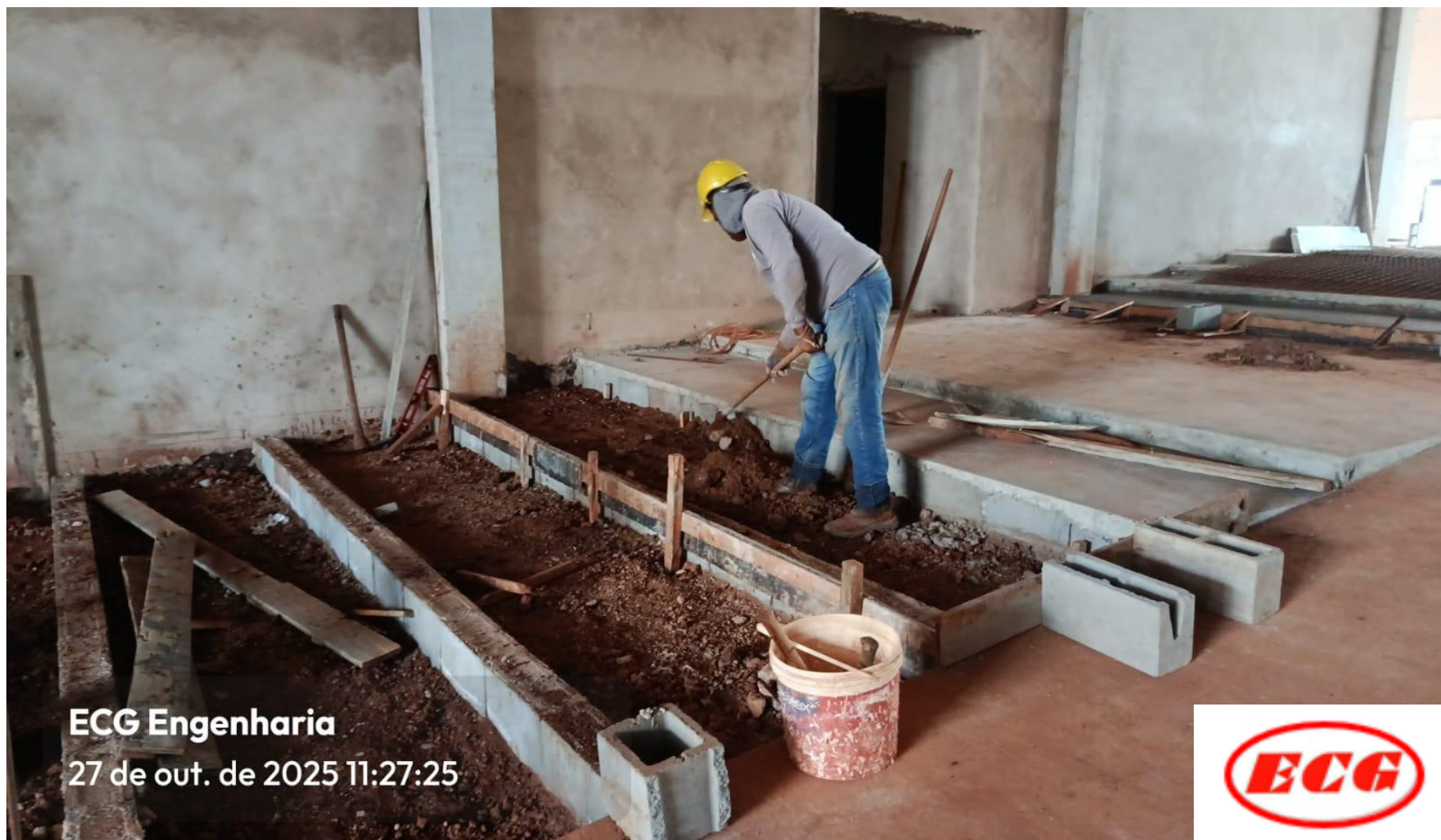
Preparação do Degrau do Plenário do Prédio em Ampliação
