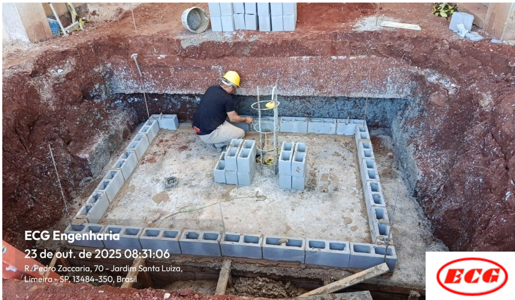
Marcação das Paredes do Poço do Elevador
