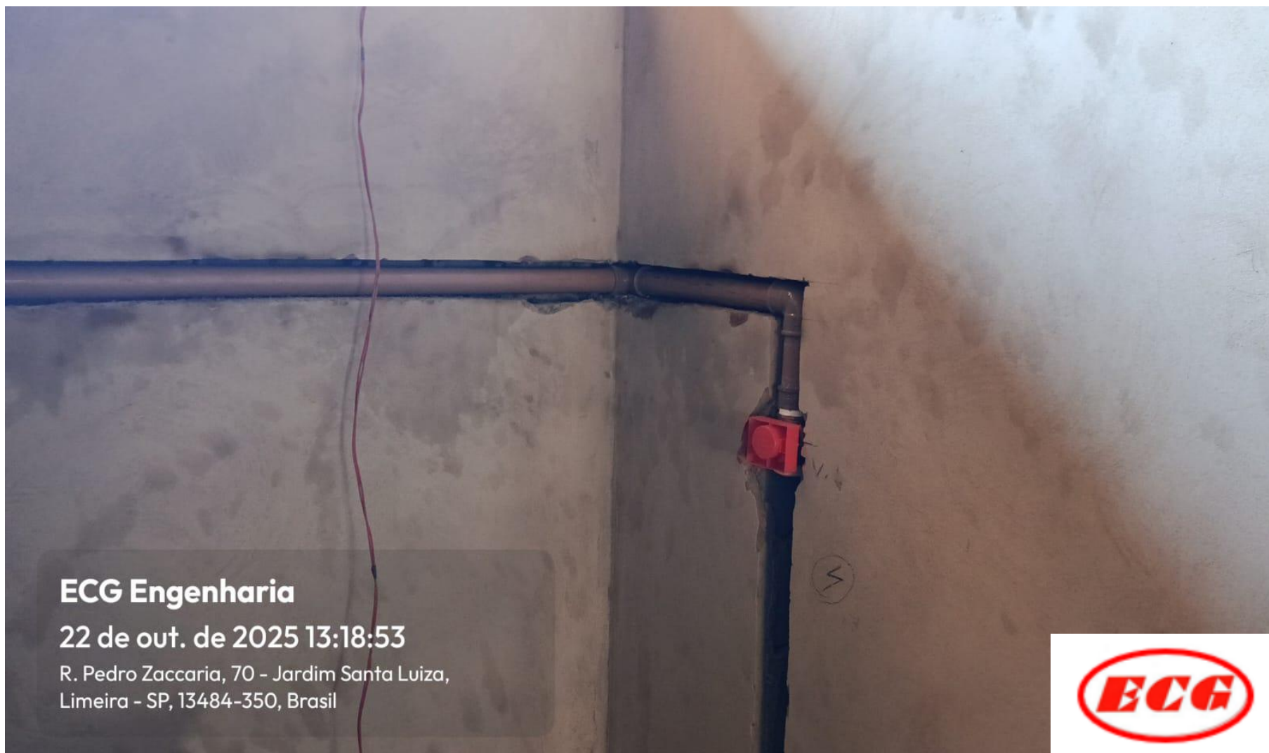
Instalação de Válvula de Descarga do banheiro do Prédio em Ampliação
