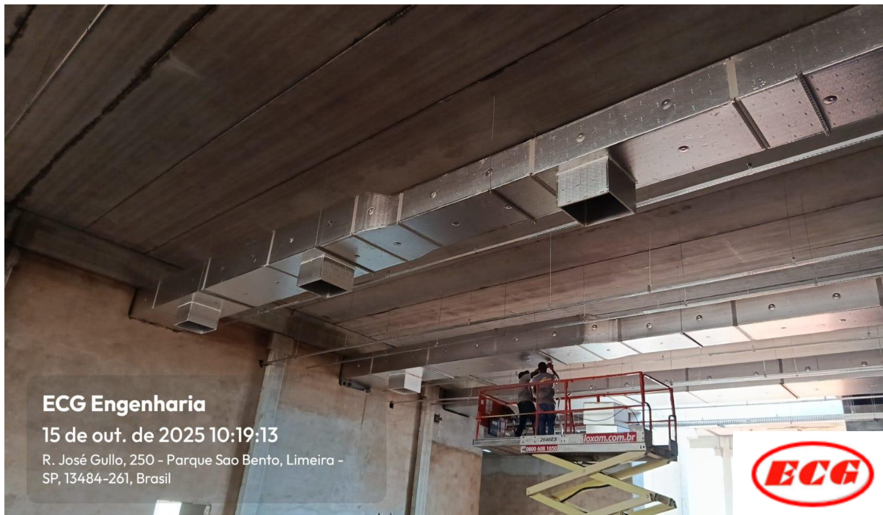
Bocal das Maquinas Cassete sendo Instalada
