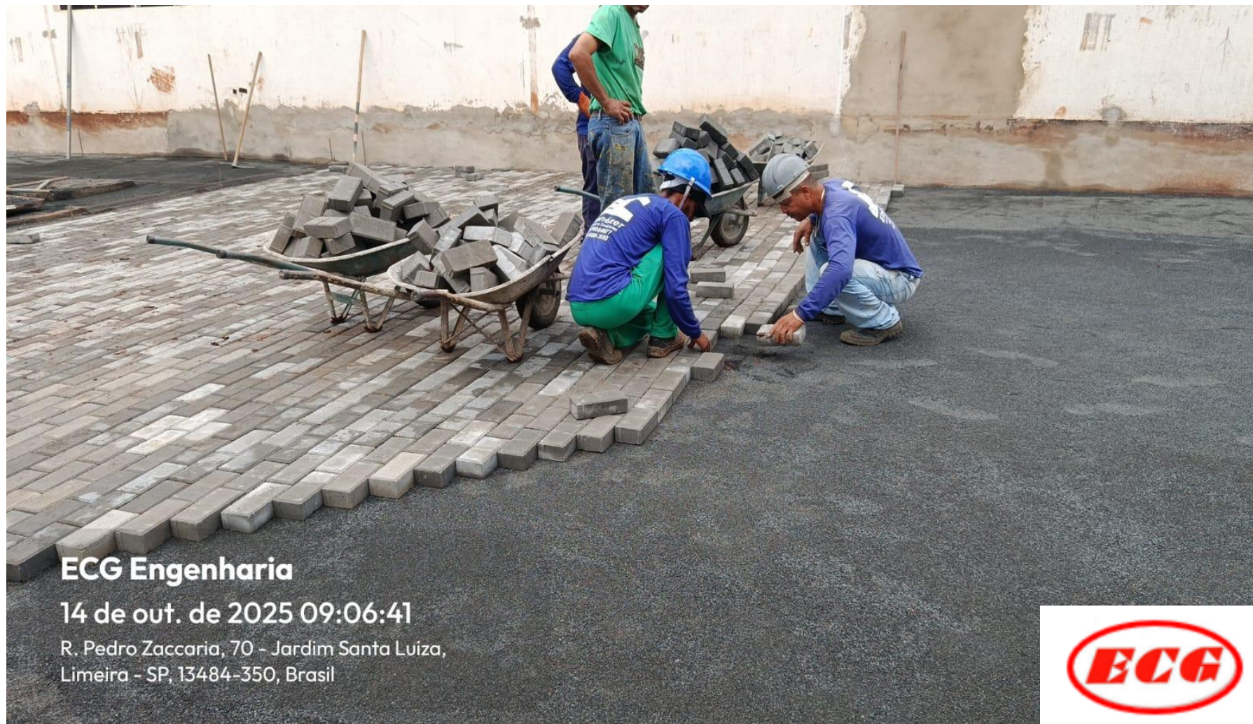
Montagem dos Intertravados do Estacionamento
