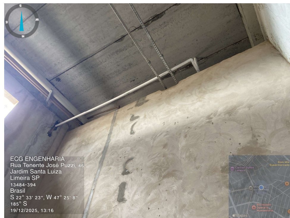
Drenos Ar-Condicionado instalados e isolados com o Elume – Prédio Ampliação.
