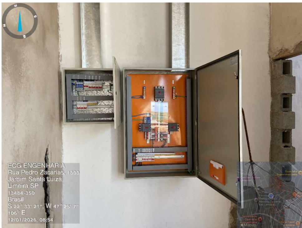
Ampliação – Montagem do quadro e toda a infra de elétrica –Pavimento Superior.
